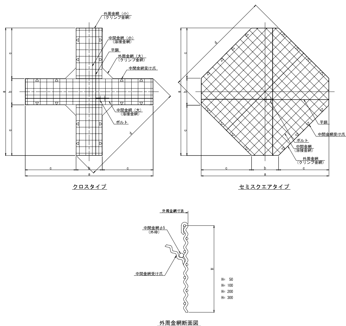
図1 ゑぶとんわくの一般的な形状
